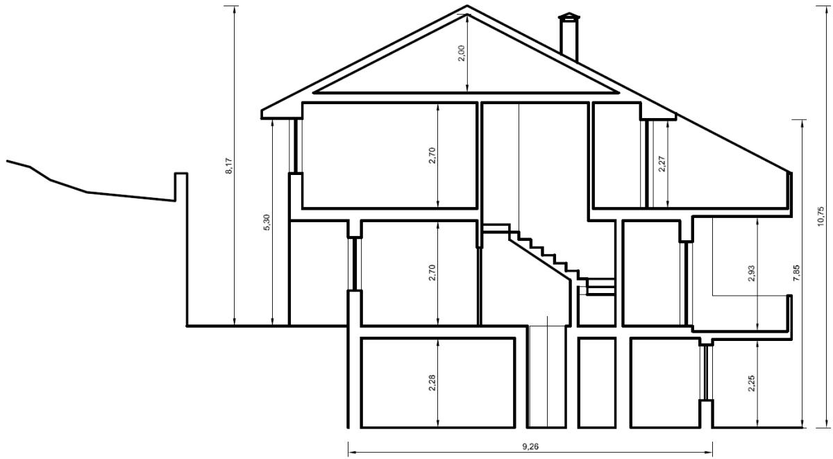
SEZIONE B-B
